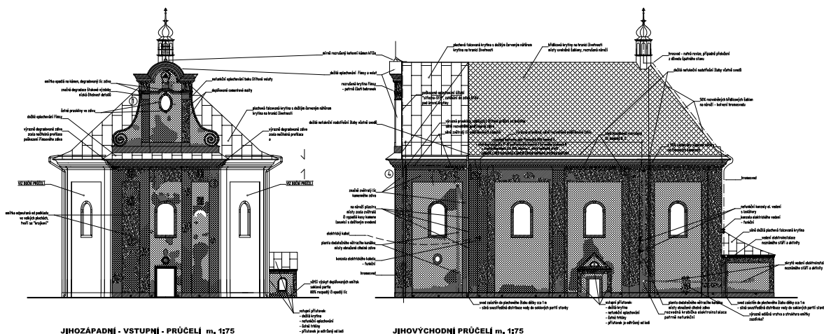
JIHOZÁPADNÍ - VSTUPNÍ - PRŮČELÍ m. 1:75
