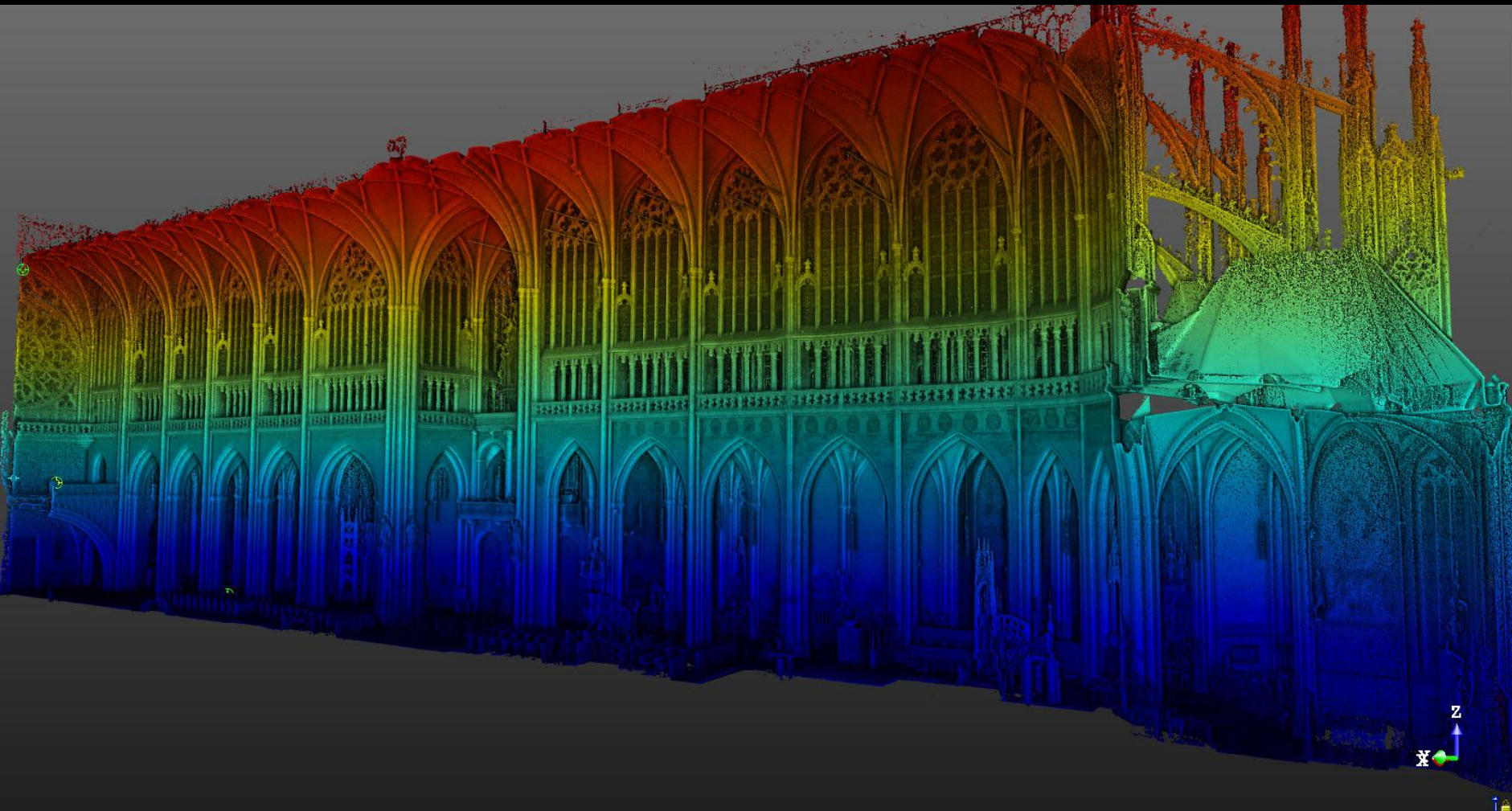
Digitalizace složité a členité architektury – katedrála sv. Víta
